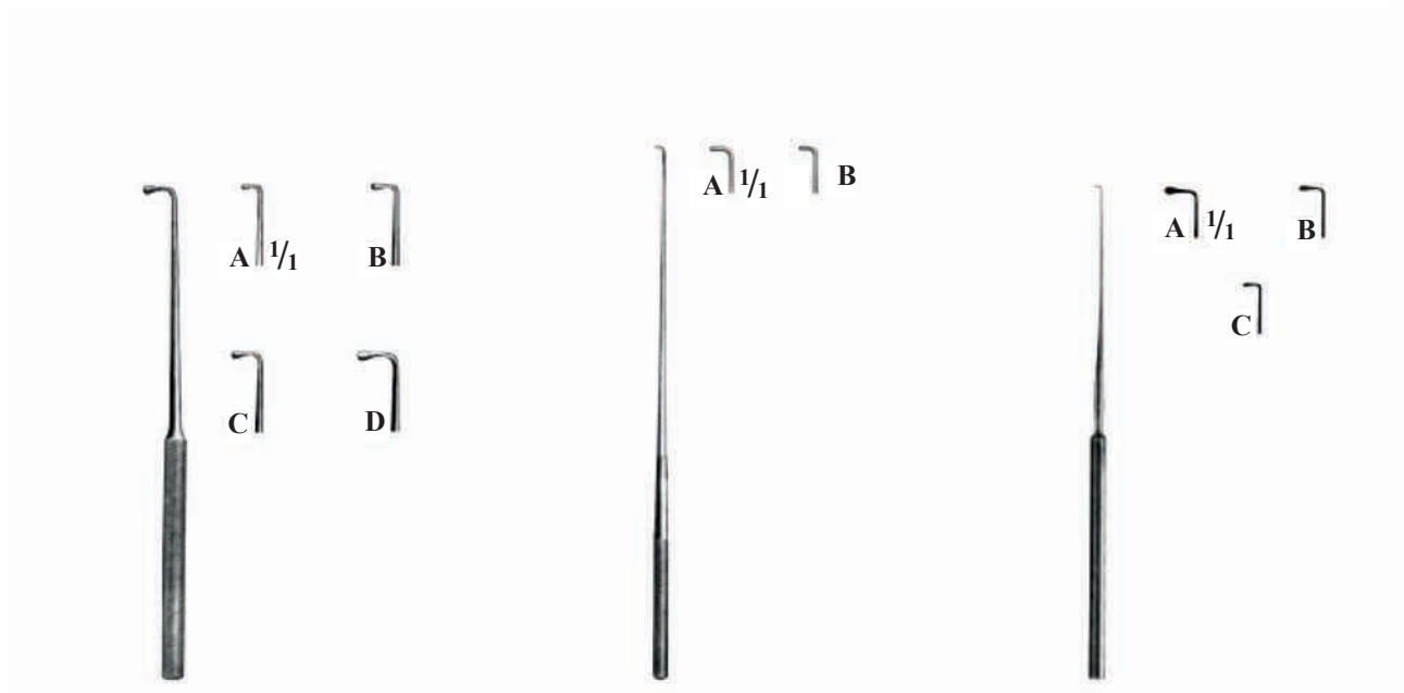
WAGENER 07-047-140 14.0 cm - A 07-048-140 14.0 cm - B 07-049-140 14.0 cm - C 07-050-140 14.0 cm - D
