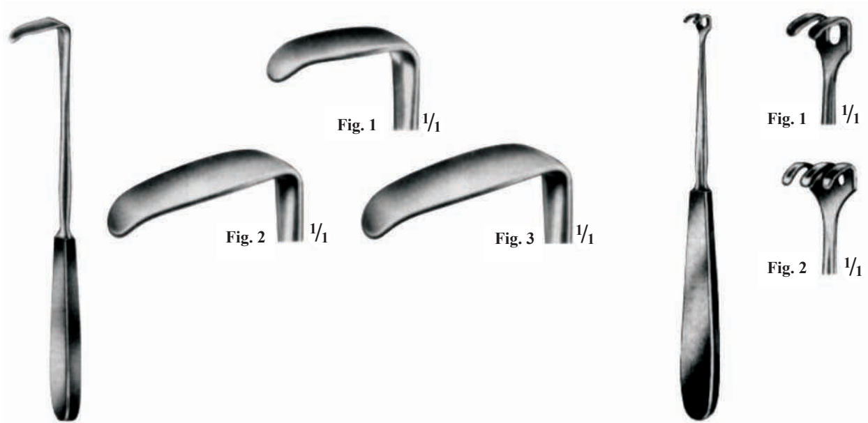
LANGENBECK 07-183-220 22.0 cm 30 x 11 mm Fig. 1 07-184-220 22.0 cm 40 x 11 mm Fig. 2 07-185-220 22.0 cm 42 x 13 mm Fig. 3
